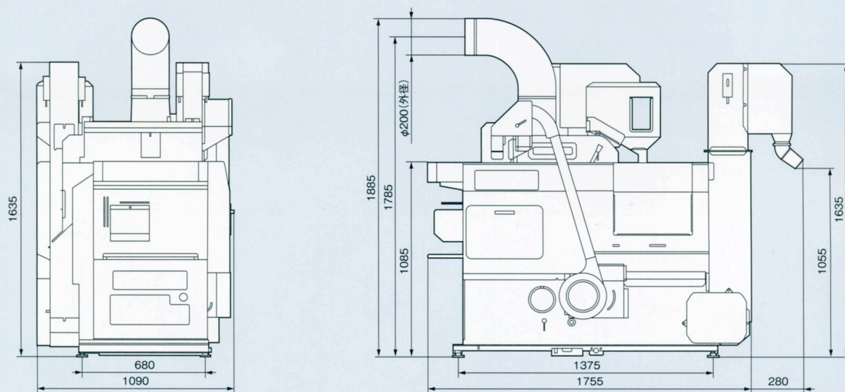
■機体寸法図(単位=mm)
